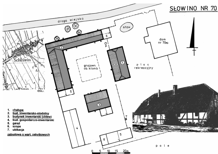
Ryc. 5. Słowo, plan zagrody chłopskiej nr 70. Oprac. W. Witek
